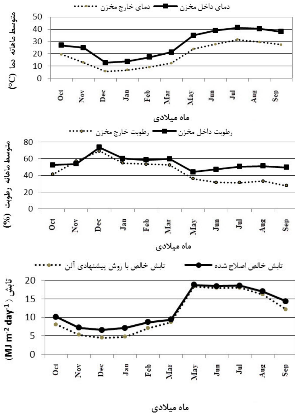
شکل ۳- روند تغییرات متوسط ماهانه پارامترهای هواشناسی (الف- دما، ب- رطوبت، ج- تابش خالص) داخل و خارج مخزن
