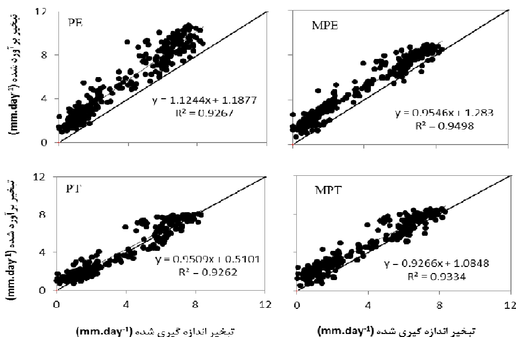
شکل ۴- پراکنش مقادیر تخمینی توسط مدل پنمن اصلاح شده (MPE)، مدل پریستلی-تیلور اصلاح شده (MPT)، مدل پنمن (PE) و مدل پریستلی-تیلور (PT) در مقابل تبخیر واقعی از مخزن (E)
