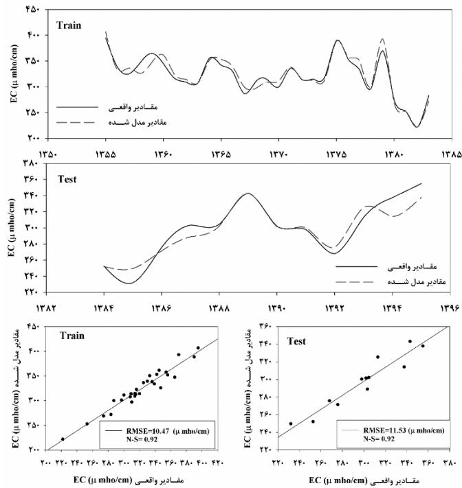
شکل ۴- نتایج بررسی میزان دقت مدل CARMA-ARCH در تخمین مقادیر EC ایستگاه هیدرومتری پی قله
