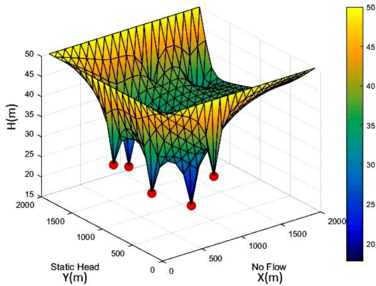
شکل ۹- میزان افت سطح آب زیرزمینی آبخوان در سناریوی ۳ (بر حسب متر)
