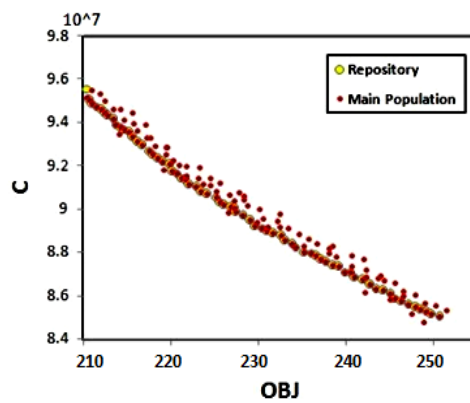
شکل ۱۰- جبهه‌ی پرتوی تولید شده برای توابع هدف توسط MOIPO در سناریوی ۱
