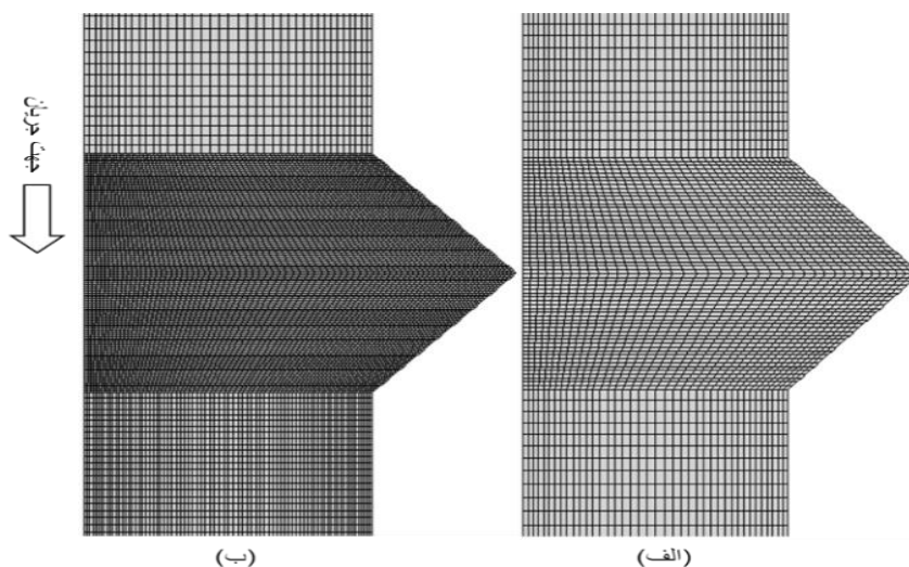
شکل ۳- اندازه‌ی شبکه محاسباتی در محدوده سرریز جانبی کنگره‌ای- (الف) ۵۰۳۲۰۰ سلول، (ب) ۲۰۱۲۴۰۰ سلول
