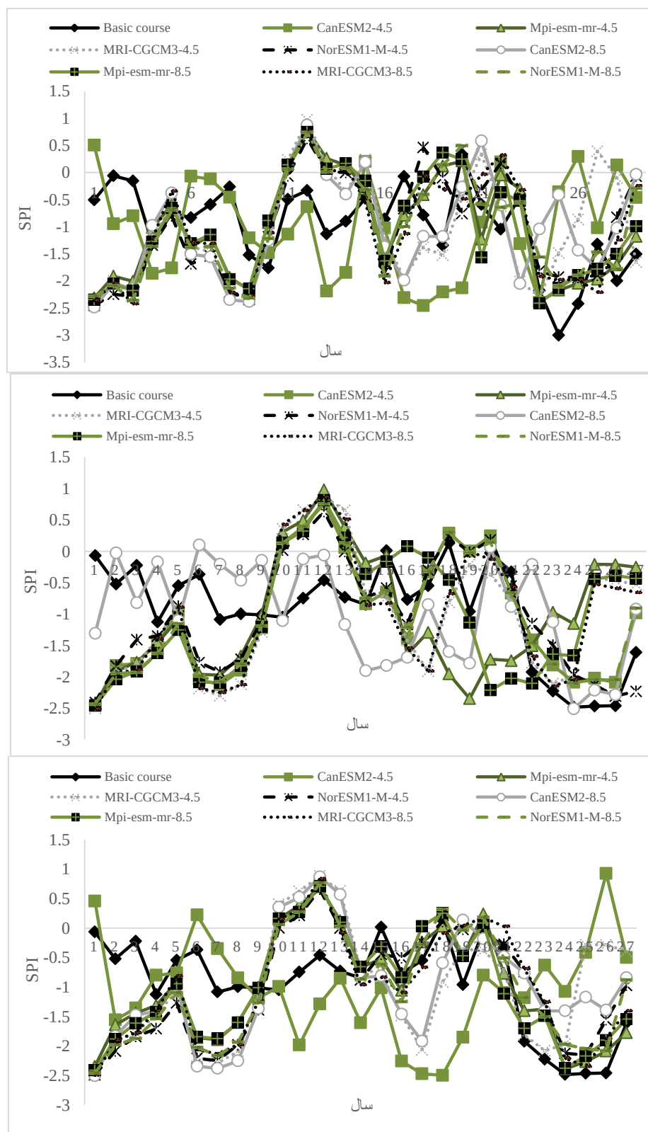
شکل ۴- مقادیر شاخص SPI ۱۲، ۲۴ و ۴۸ ماهه (به ترتیب از بالا به پایین) برای دو دوره آتی نزدیک (۲۰۱۵-۲۰۴۵) (سمت چپ) و دوره آتی دور (۲۰۷۵-۲۰۴۵) (سمت راست) و مدل های GCM و دو سناریو RCP4.5 و RCP8.5
