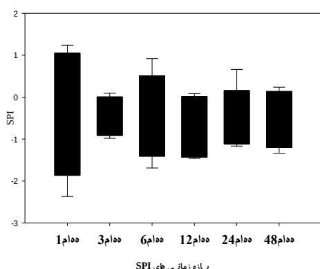
شکل ۵- دامنه تغییرات بازه زمانی‌های SPI برای دوره آتی (۲۰۴۵-۲۰۷۵) (بالا) و (۲۰۷۵-۲۰۴۵) (پایین) برای سناریو RCP4.5 (راست) و سناریو RCP8.5 (چپ)
