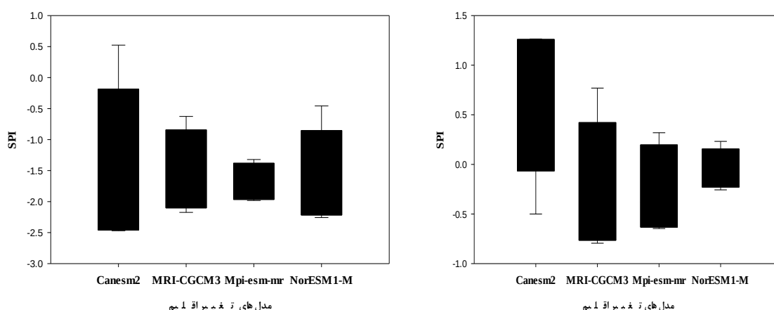
شکل ۶- دامنه تغییرات SPI کوتاه (راست) و طولانی (چپ) مدت برای مدل‌های تغییر اقلیم
