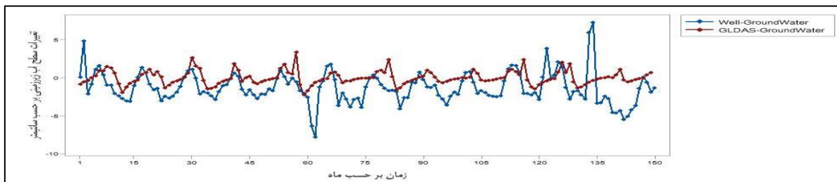
شکل ۱۱- مقایسه تغییرات سطح آب زیرزمینی با استفاده از داده‌های مشاهداتی (چاه‌ها) و GLDAS در پیکسل به طول جغرافیایی ۵۷/۵ الی ۵۸/۵
