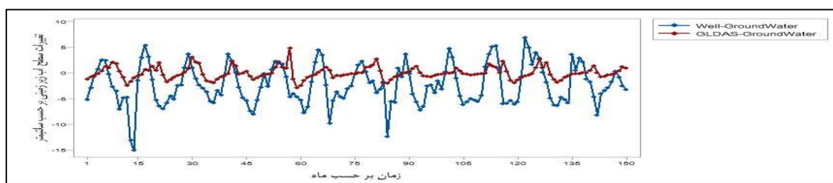
شکل ۱۳- مقایسه تغییرات سطح آب زیرزمینی با استفاده از داده‌های مشاهداتی (چاه‌ها) و GLDAS در بیکسل به طول جغرافیایی ۵۸/۵ الی ۵۹/۵
