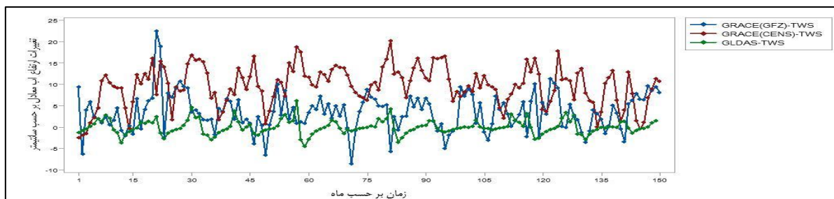
شکل ۵- مقایسه مقادیر TWS یا EWH داده‌های مراکز پردازش GFZ و CENS و GLDAS در پیکسل به طول جغرافیایی ۵۸/۵ الی ۵۹/۵
