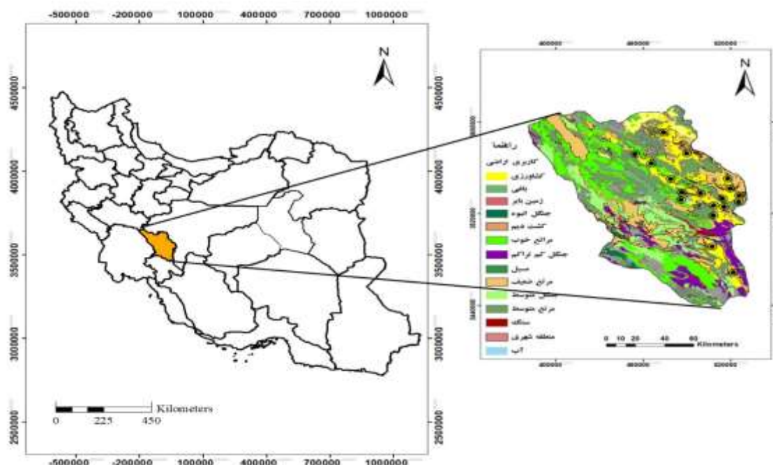
شکل ۱- منطقه مورد مطالعه و محل چاه‌های انتخاب‌شده
