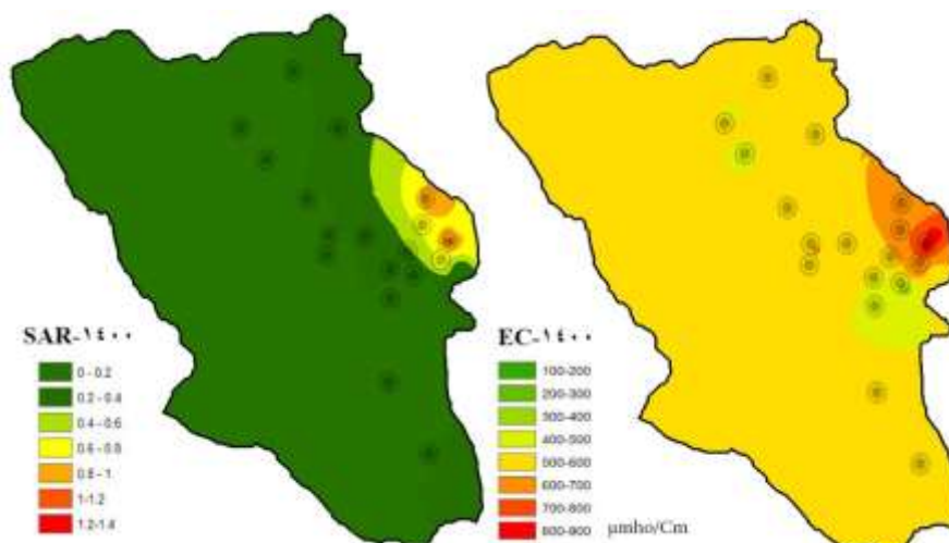
شکل ۵- پهنه‌بندی منطقه از نظر SAR و EC در سال ۱۴۰۰
