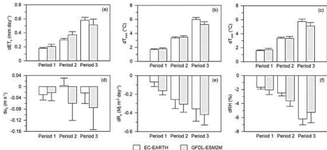
شکل ۶- نمودارهای مقایسه میانگین و انحراف معیار تفاضل مقادیر میانگین بلندمدت سالانه ET_0 (a)، دمای بیشینه (b)، دمای کمینه (c)، سرعت باد (d)، تابش خورشیدی (e) و رطوبت نسبی (f) دوره‌های آینده (۲۰۱۱-۲۰۴۰ (Period 1)، ۲۰۴۱-۲۰۷۰ (Period 2) و ۲۰۷۱-۲۱۰۰ (Period 3)) نسبت به مقادیر متناظر آنها در دوره تاریخی (۱۹۷۶-۲۰۰۵) برای یاخته‌های مدل‌های EC-EARTH و GFDL-ESM2M در منطقه مورد مطالعه
