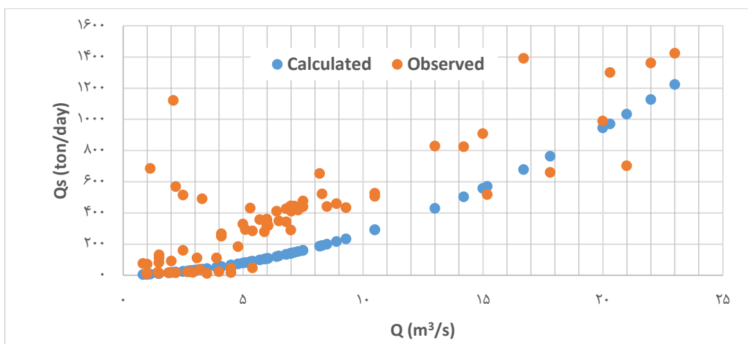
شکل ۸- تغییرات مقدار بار کف بر حسب مقدار دبی جریان در ماه‌های مختلف سال با استفاده از رابطه بگنولد
