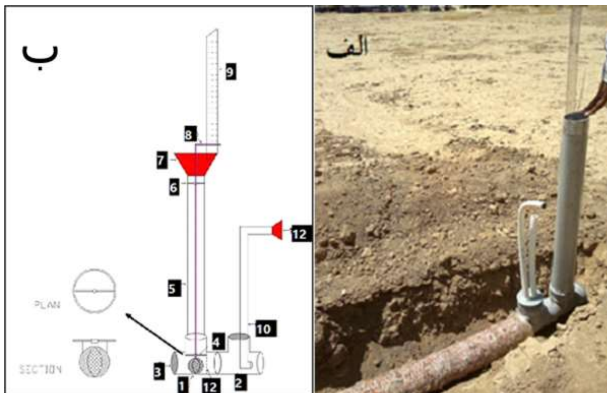
شکل ۱- نمای کلی لوله سوراخ‌دار و شناور نصب‌شده داخل لوله تغذیه. در این شکل: (الف) تصویر لوله استفاده‌شده در آزمایش، (ب) ۱- نشان‌دهنده شناور کروی، ۲- سهراهی UPVC، ۳- درپوش UPVC، ۴- نگاه‌دارنده متحرک شناور، ۵- لوله غیر مشبک UPVC با قطر داخلی ۹۰ میلی‌متر (لوله تغذیه)، ۶- نگاه‌دارنده میله هادی شناور، ۷- آبیگر لوله، ۸- نشانگر خط‌کش، ۹- خط‌کش مدرج، ۱۰- لوله ۵ لایه با قطر داخلی ۳۲ میلی‌متر، ۱۱- اتصال رزوه‌دار و ۱۲- سیم‌های حائل برای جلوگیری از انحراف شناور و گیر کردن آن در موقع بالا آمدن است.
