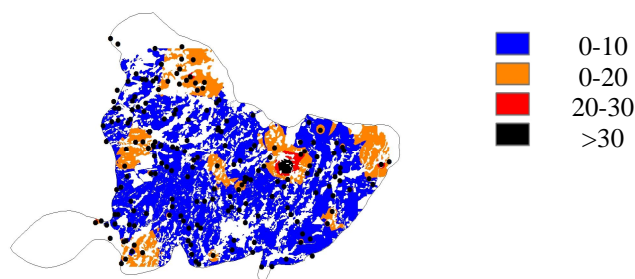
شکل 6 - نقشه درصد خطای مطلق مدل برای پیش بینی عملکرد
