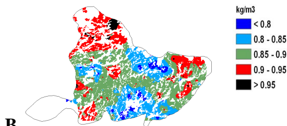
شکل 7 - بهره‌وری آب اندازه‌گیری شده مبتنی بر مصرف آب (A) و تعرق (B)
