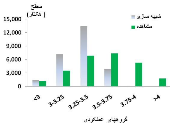
نمودار 2- سطح زیر کشت واقعی و شبیه‌سازی شده توسط مدل در گروه‌های مختلف عملکردی (کیلوگرم در هکتار)
