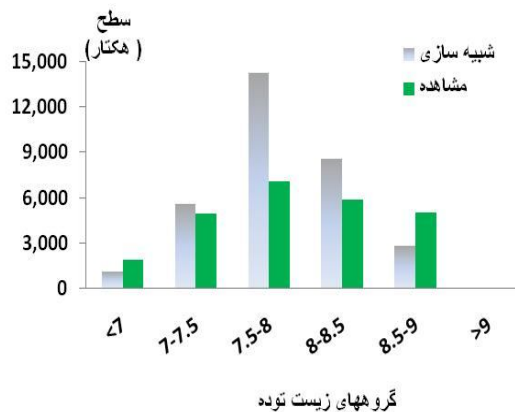
نمودار 4- سطح زیر کشت برنج واقعی و شبیه‌سازی شده توسط مدل در گروه‌های مختلف زیست توده (کیلوگرم در هکتار)
