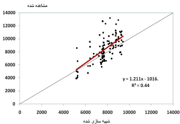
نمودار 5- مقایسه زیست توده برنج مشاهداتی و شبیه‌سازی شده توسط مدل در سطح وسیع (کیلوگرم در هکتار)
