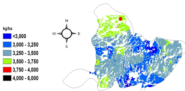
شکل 3 - نقشه عملکرد شبیه‌سازی شده توسط مدل
