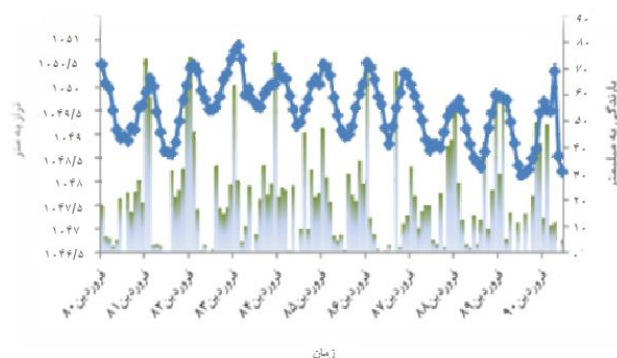
شکل 5- هیدروگراف واحد دشت بجنورد طی دوره مدل‌سازی (1380-1390)
