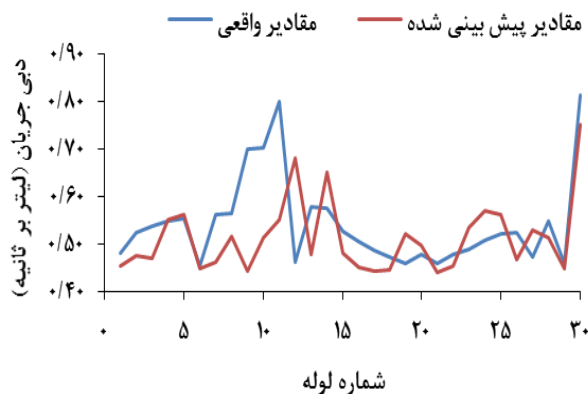
شکل ۵- مقایسه مقادیر محاسبه شده و پیش‌بینی شده دبی جریان در ناحیه ۱
