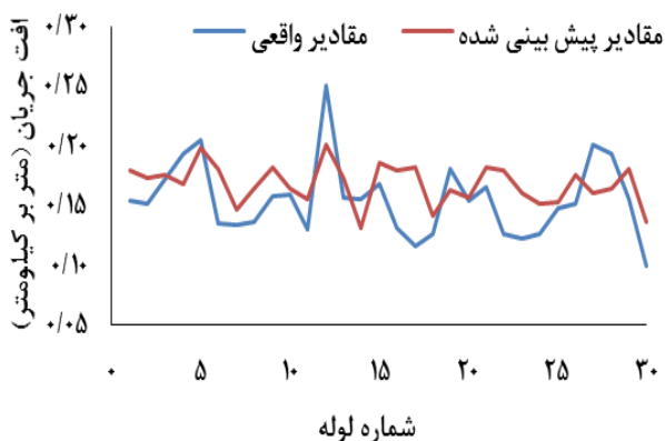
شکل ۷- مقایسه مقادیر محاسبه شده و پیش‌بینی شده افت جریان در ناحیه ۱
