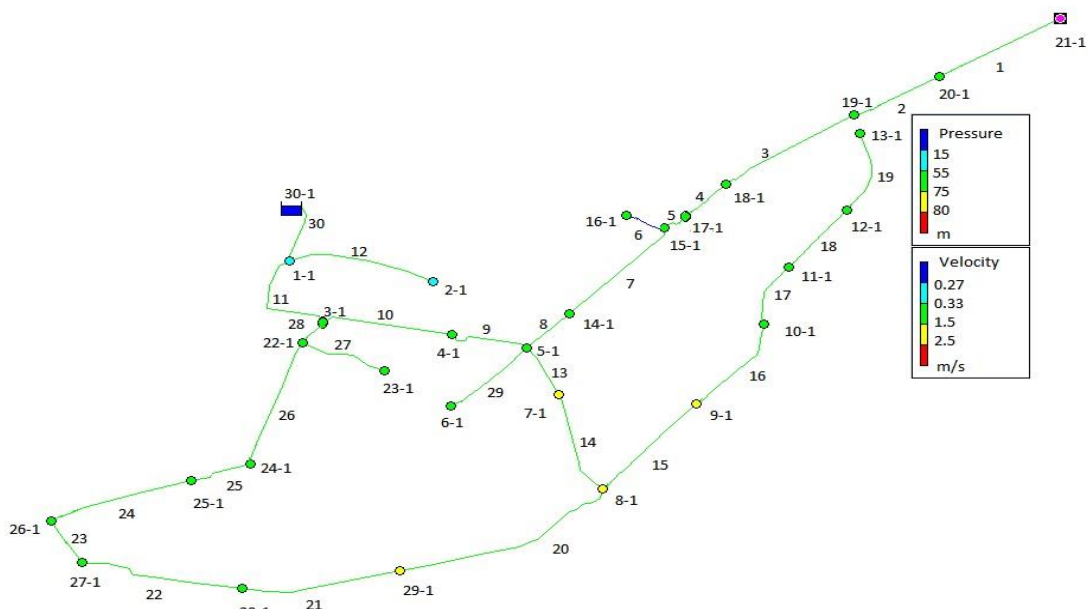
شکل ۳- فشار در گره ها و سرعت در لوله ها در ناحیه فشاری ۱
