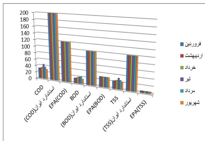
شکل ۲- مقادیر متوسط پارامترهای COD، BOD 5 و TSS پساب تصفیه‌خانه فاضلاب تفرش در مقایسه با استاندارد مصارف کشاورزی
