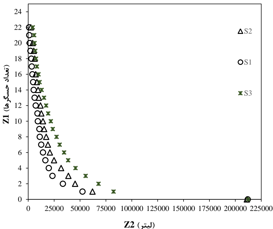
شکل ۲- پارتوی بهینه محل حسگرها بر اساس خسارت بحرانی (حجم آب آلوده) به ازای تعداد حسگرها
