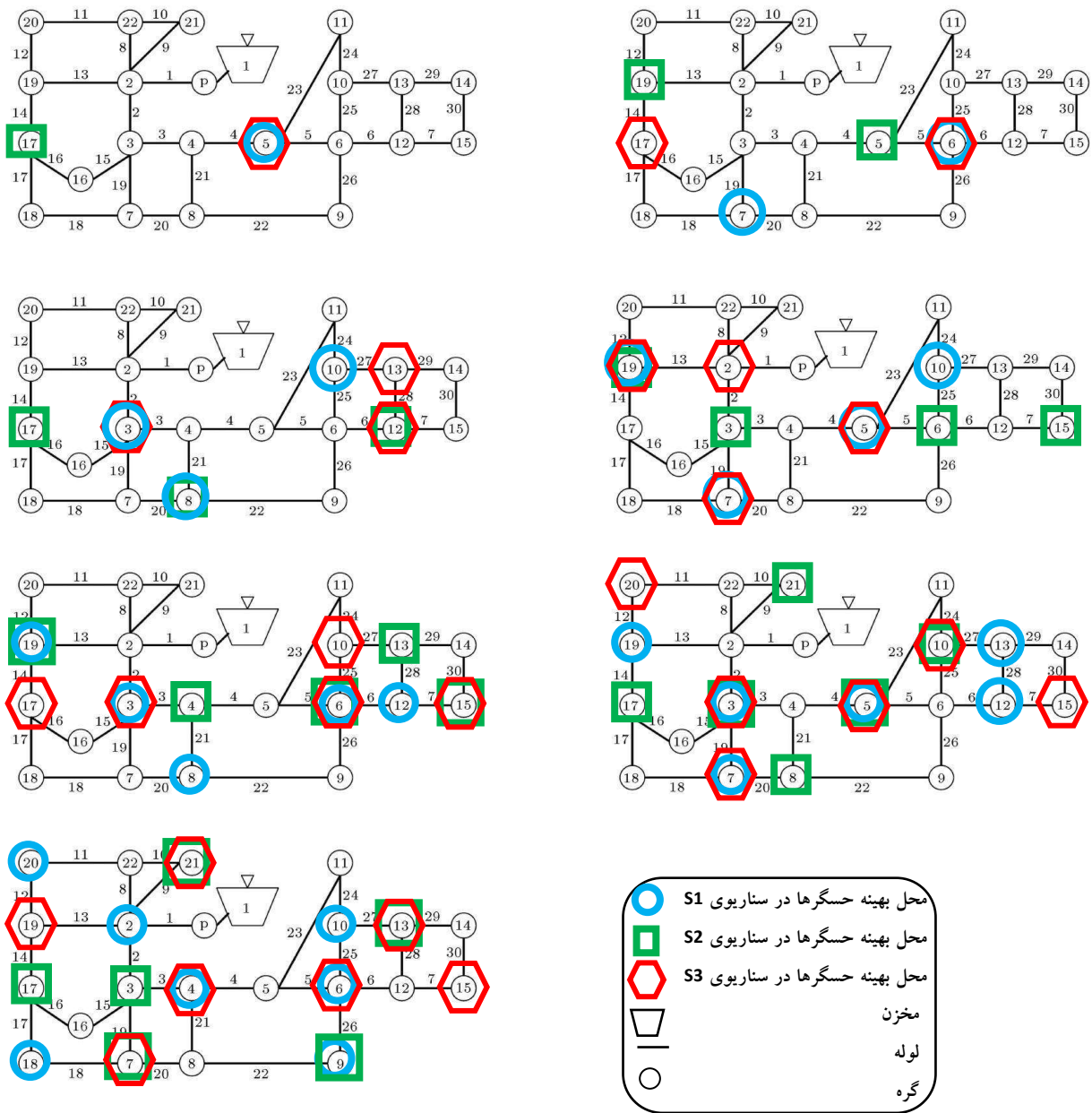
شکل ۴- محل بهینه حسگرها به ازای ۱ تا ۷ حسگر در شبکه مطالعاتی
