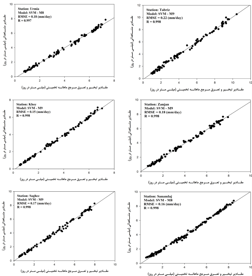
شکل ۴- نمودارهای پراکندگی مقادیر مشاهده‌ای و تخمینی تبخیر-تعرق ماهانه گیاه مرجع در بهترین حالت مدل SVM برای ایستگاه‌های منتخب شمال غرب ایران
