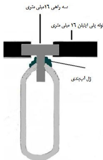
شکل 1- کوزه رسی مخصوص آبیاری و ساختار آن
