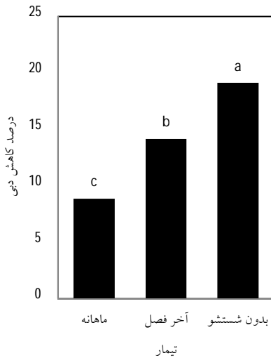
شکل 12- ضریب تغییرات دبی در دوره‌های مختلف شستشو
