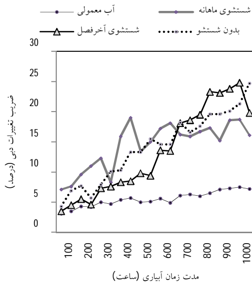
شکل 5- مقادیر ضریب تغییرات دبی قطره چکان کرونا در زمان‌های مختلف در شروع آزمایش
