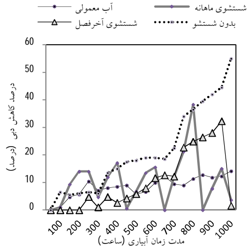
شکل 1- روند تغییرات درصد کاهش دبی قطره‌چکان میکروفلاپر
