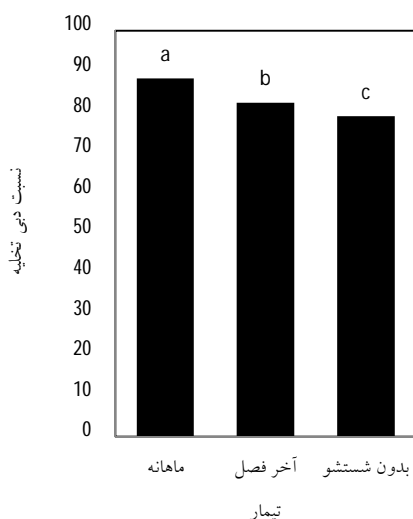
شکل 16- نسبت دبی تخلیه در دوره‌های مختلف شستشو
