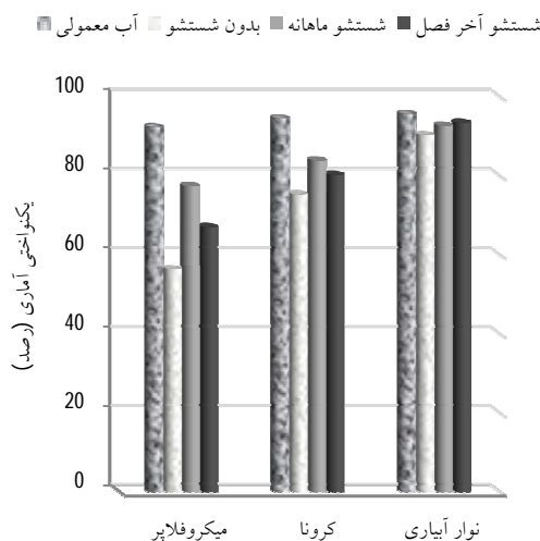
شکل 8-مقادیر یکنواختی آماری قطره‌چکان‌ها در انتهای دوره‌ی آزمایش
