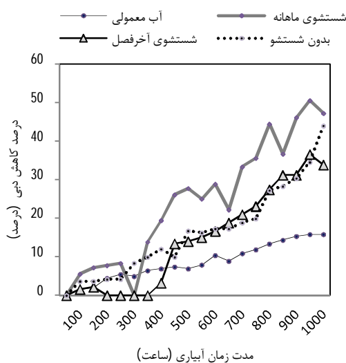
شکل 2- روند تغییرات درصد کاهش دبی قطره‌چکان کرونا
