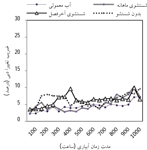
شکل 6- مقادیر ضریب تغییرات دبی نوار آبیاری در زمان‌های مختلف در شروع آزمایش
