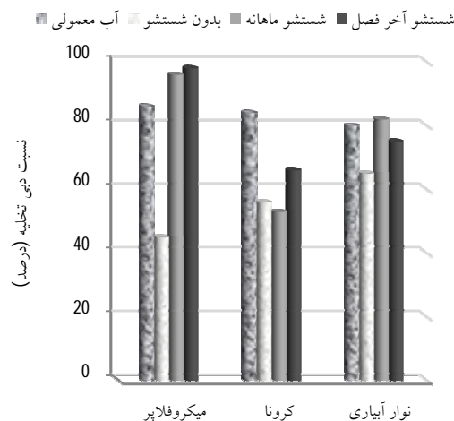
شکل 7- مقادیر نسبت دبی تخلیه قطره‌چکان‌ها در انتهای دوره آزمایش
