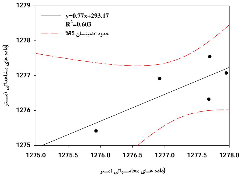
شکل 5- نتایج صحت سنجی مدل آرما جهت پیش بینی تراز سطح آب دریاچه
