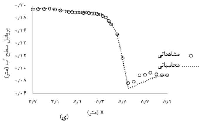
شکل ۱۴ - پروفیل سطح آب در Y=0.3 \text{ m} (مدل A): الف؛ Q=0.01 \text{ m}^3/\text{s} ؛ ب؛ Q=0.0145 \text{ m}^3/\text{s} ؛ ج؛ Q=0.0185 \text{ m}^3/\text{s} ؛ د؛ Q=0.021 \text{ m}^3/\text{s} ؛ ه؛ Q=0.0255 \text{ m}^3/\text{s} ؛ ی؛ Q=0.03 \text{ m}^3/\text{s}
