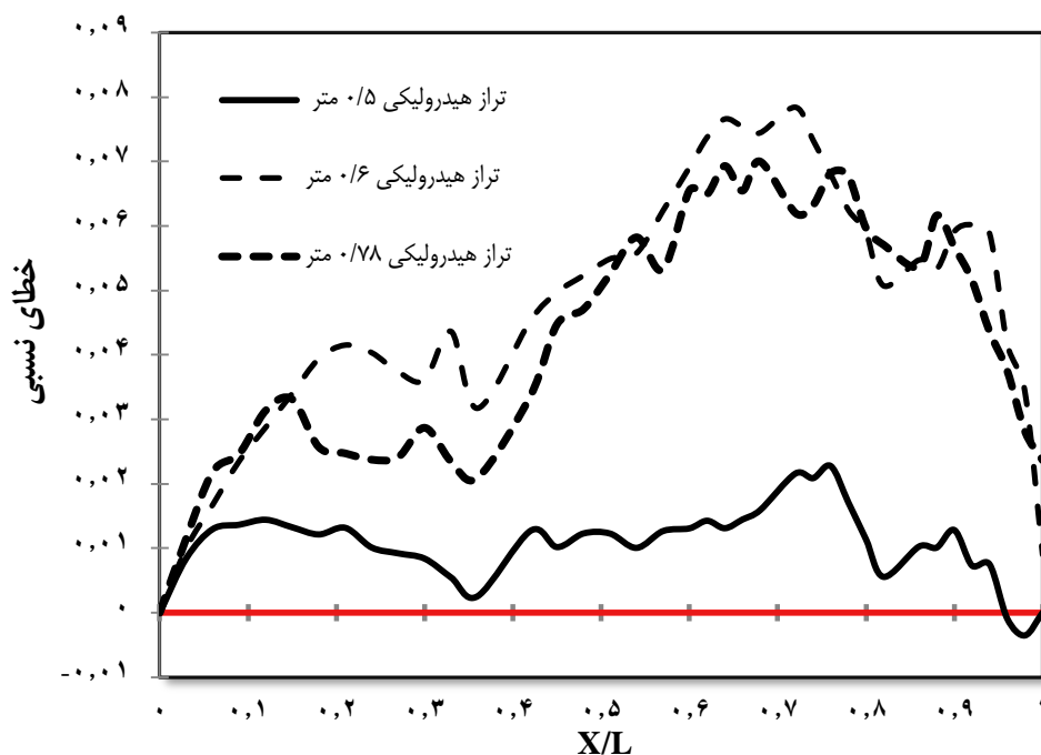
شکل ۶- خطای نسبی تخمین عمق نتایج آزمایشگاهی و رابطه تحلیلی چاپمن (1956) در طول فلوم
