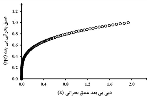
شکل ۱۱- دبی بی بعد در برابر عمق بحرانی بی بعد
