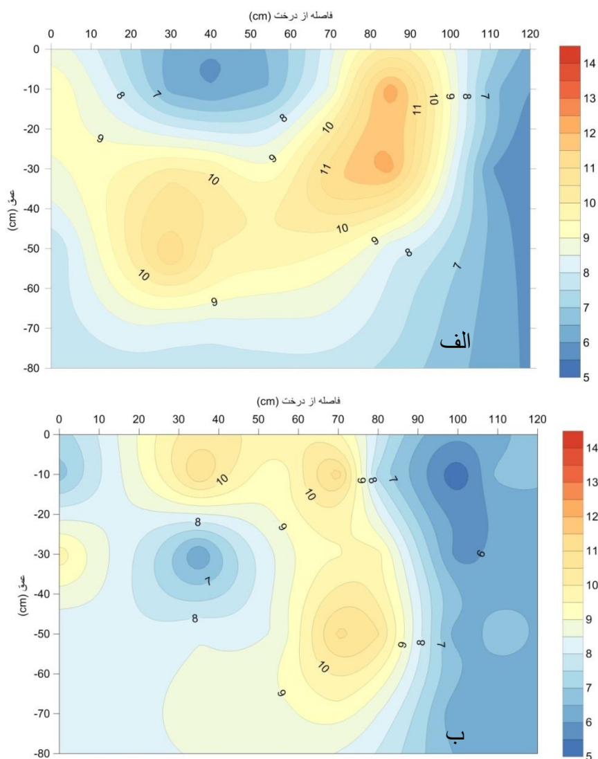
شکل ۲- تغییرات توزیع شوری خاک در دو سامانه آبیاری قطره‌ای سطحی (الف) و زیرسطحی (ب)
