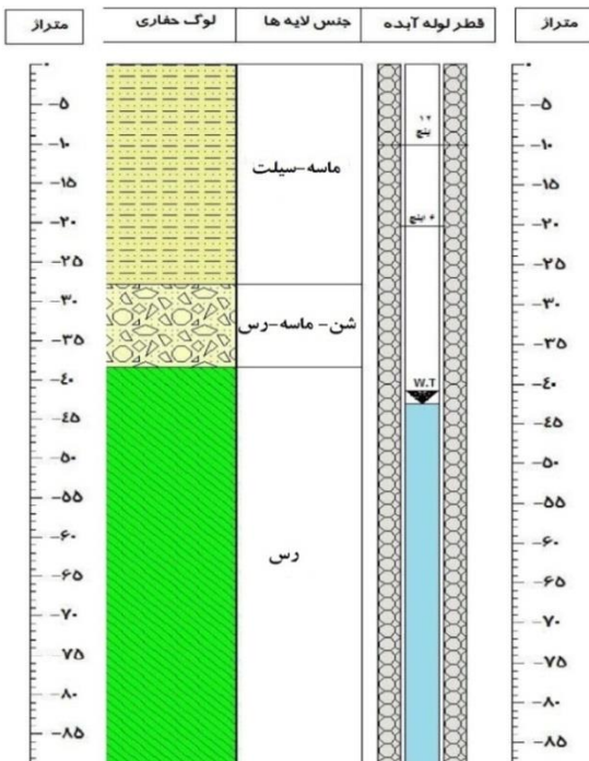
شکل ۷- تغییرات سطح آب زیرزمینی در چاه پیزومتری شماره ۹
