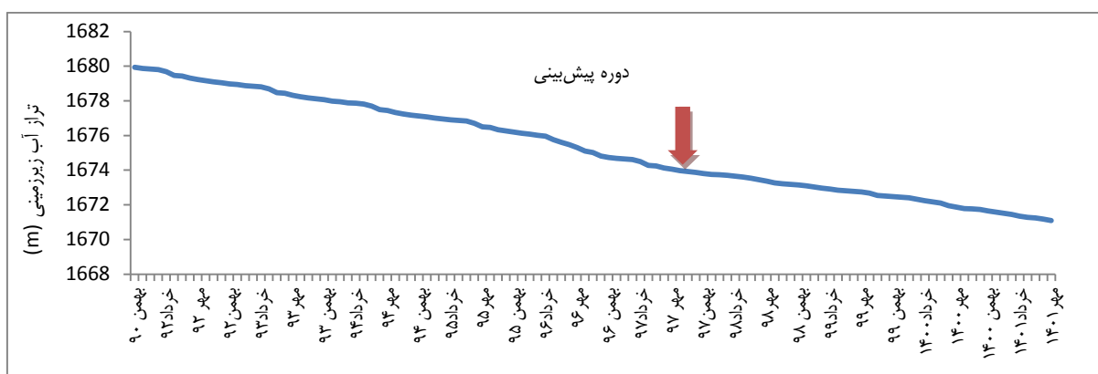
شکل ۱۴- نمودار افت طی دوره پیش‌بینی در پیزومتر شماره ۲ دشت سیرجان
