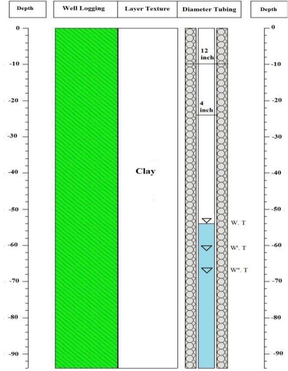
شکل ۴- تغییرات سطح آب زیرزمینی در چاه پیزومتری شماره ۳
