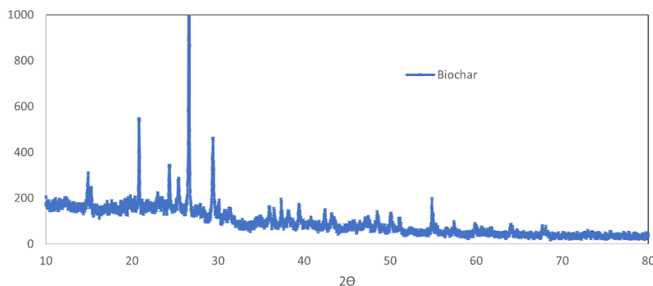
شکل ۵- آنالیز پراش اشعه ایکس (XRD) جاذب بیوچار
