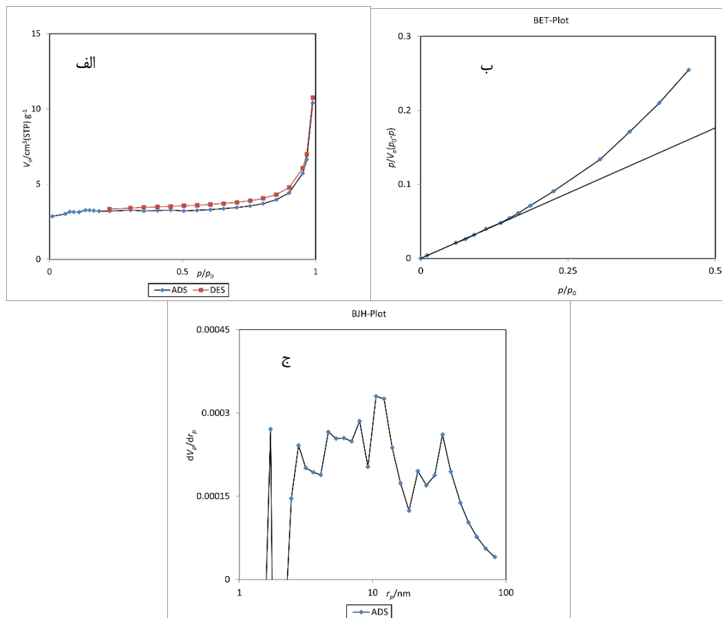
شکل ۱- پلات های الف: ADS-DES، ب: BET و ج: BJH جاذب بیوچار
